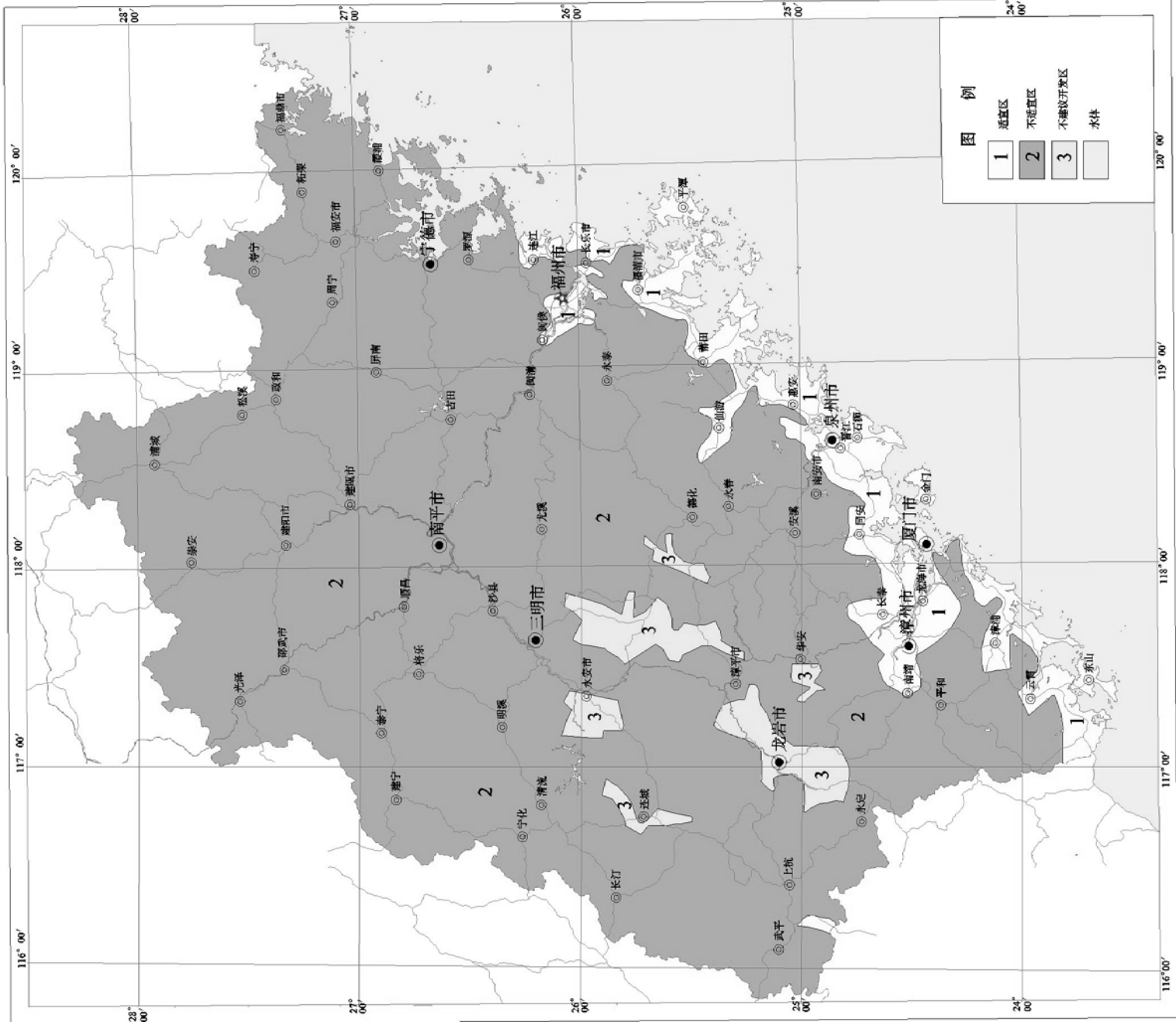
图 D-1 福建省地下水热源泵适宜性分区图
